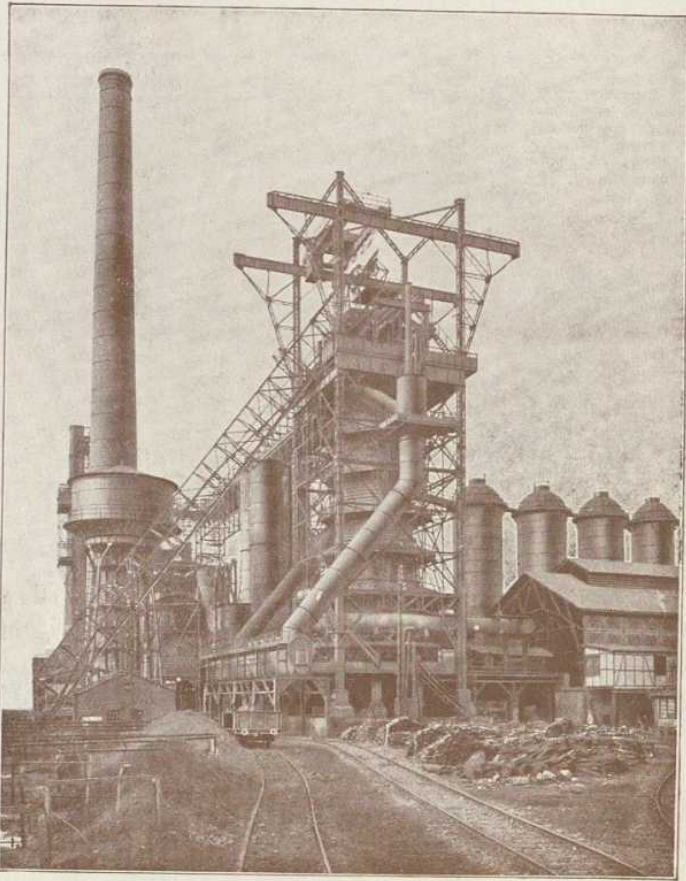
Hochöfen der Henrichshütte.
